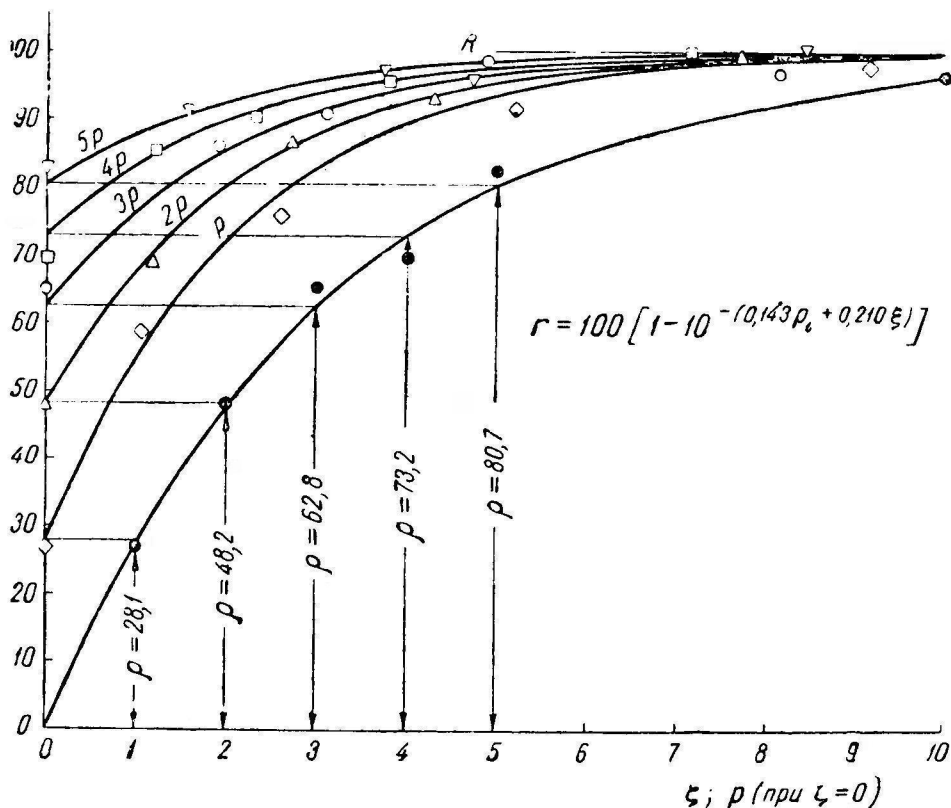
Рис. 6. Зависимость размеров рациона от плотности и агрегатности пищевого материала в системе Syrpinus carpio → Chironomidae (обозначения те же, что на рис. 5)
