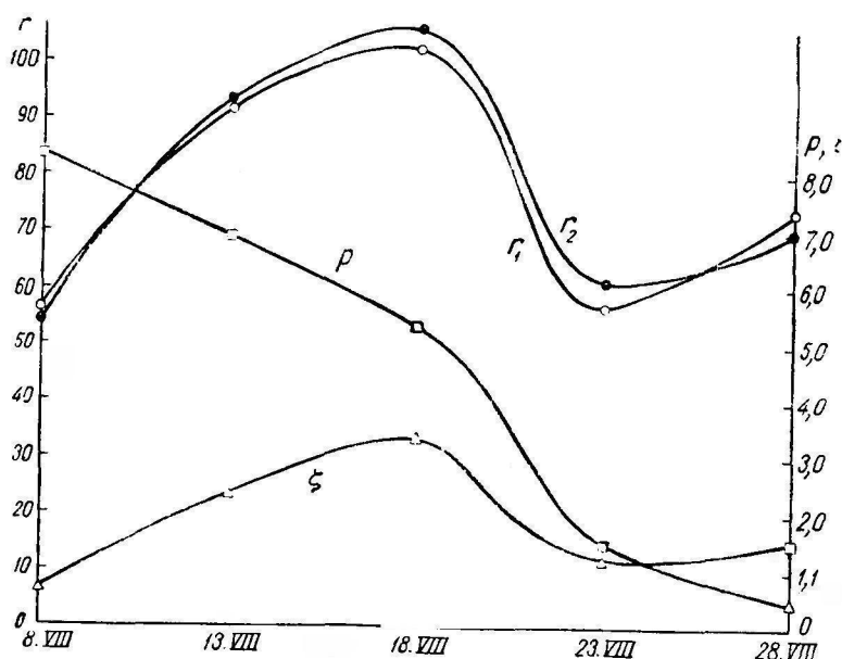
Рис. 8. Изменения средней плотности бентоса, его агрегатности и размеров рационов (найденных эмпирически ( r_1 ) и вычисленных ( r_2 )).
