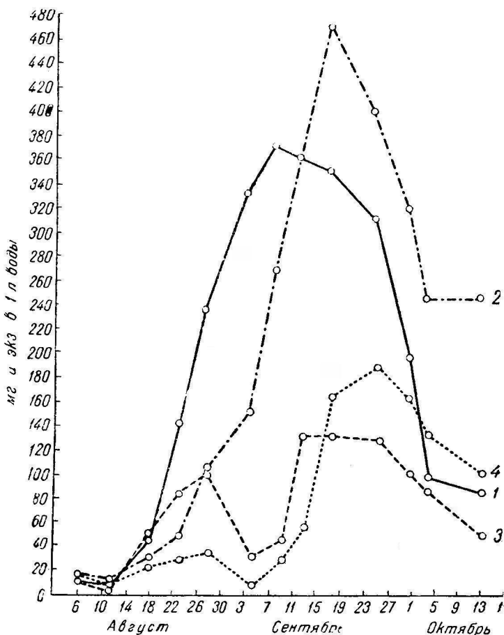
Рис. 1. Развитие популяции Daphnia magna в опытном и контрольном водоемах. 1 — плотность в опытном водоеме, 2 — биомасса в опытном водоеме, 3 — плотность в контрольном водоеме, 4 — биомасса в контрольном водоеме
