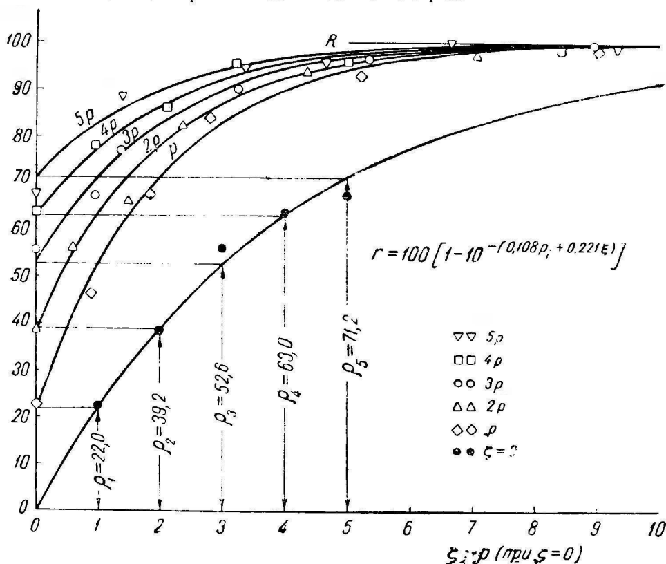
Рис. 5. Зависимость размеров рациона от плотности и агрегатности пищевого материала в системе Sucripus caprio → не живой корм
