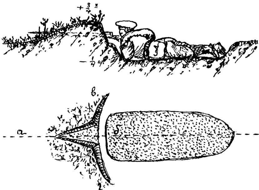
Рис. № 10. Маска изъ дерна (профиль и планъ). Дернъ надрѣзывается по линіямъ: аб и гв, затѣмъ углы дернинъ приподнимаются.
