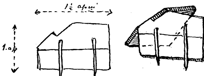
Рис. № 8. Треугольная бойница. а) Обрубковъ доски отдѣльно. б) Два обрубка вмѣстѣ.
