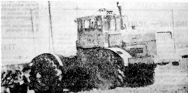
Трактор Т-150 К. Эта техника в наш район начала поступать в начале восьмидесятых годов. На ней до сих пор пахут, культивируют... И хотя многие ругают эти тракторы за то, что они уплотняют землю, без этого трактора-труженика сегодня пока еще не обойтись.
