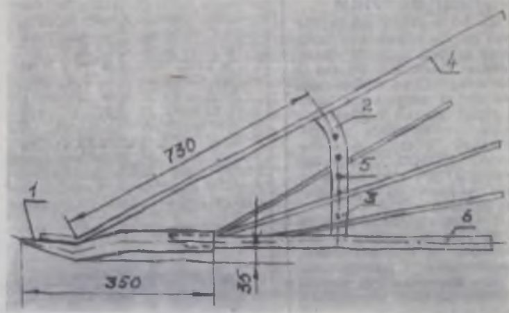
Приспособление для уборки полеглого и скрученного льна: 1 — наконечник-удлинитель; 2 — сектор; 3 — стойка; 4 — прутки-разделители стеблей; 5 — стяжной болт; 6 — делитель теребильного аппарата.
