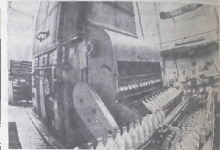
Башенный автомат непрерывного действия стерилизации молока на Можайском заводе.
