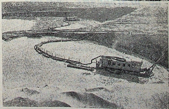
ТУРКМЕНСКАЯ ССР. В Тахта-Базарском районе Марыйской области, на реке Мургаб, ведется сооружение Сары-Язникского водохранилища, первая очередь которого вместит 660 миллионов кубометров воды.
