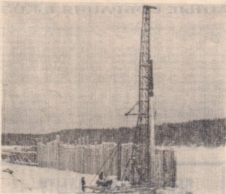
Осенью прошлого года на берегу Сухоны, в районе Крестовки, началось строительство Тотемского речного причала. По лицевой стороне причальной линии забито 160 двенадцатиметровых железобетонных свай, ведутся забивка свай боковых стенок и другие работы.
