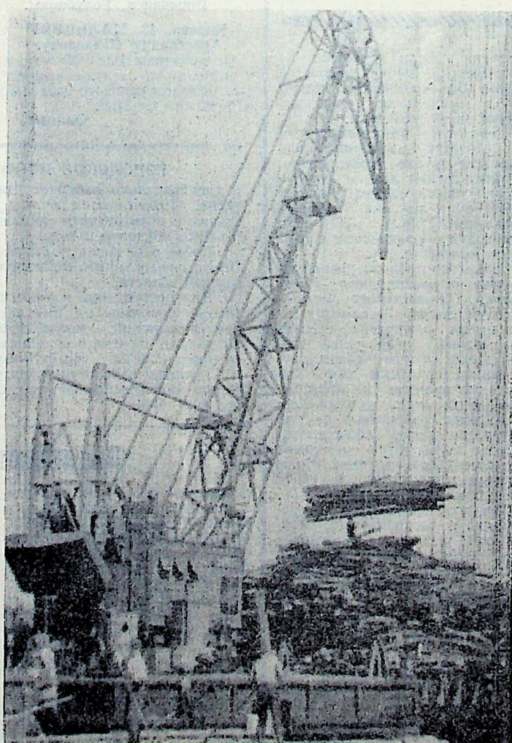
На снимке: бригада сплавщиков ведет погрузку древесины в баржу краном КПЛ-5-30. Управляет краном С. Н. Волохов. Он знает свое дело, умело подводит стрелу к древесине и быстро поднимает ее на баржу.
