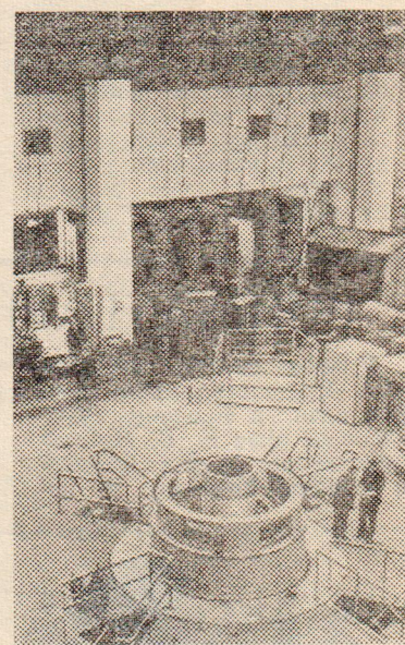
Гидростанция у Дивных гор на Енисее достигла мощности в шесть миллионов киловатт. В конце декабря пущен последний 12-й агрегат.
