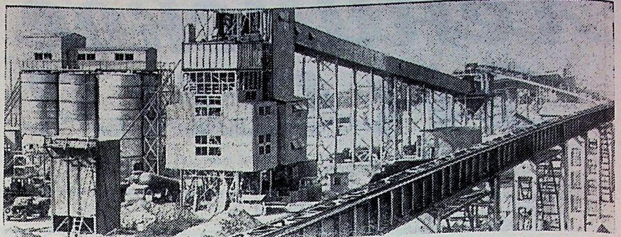
На строительстве Ретарского алюминиевого завода — первенца цветной металлургии Таджикистана — горячая пора. Завершается возведение подсобных предприятий, сооружаются производственные корпуса. Первый
