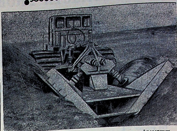
Промышленность освоила серийный выпуск фрезерных канавкопателей КФН-1200, которые применяются при осушении болот. Машина оставляет за собой канаву глубиной до 1,2 метра. Она может заменить четыре ковшевых экскаватора. При этом себестоимость выемки одного кубометра грунта снижается до трех копеек.
