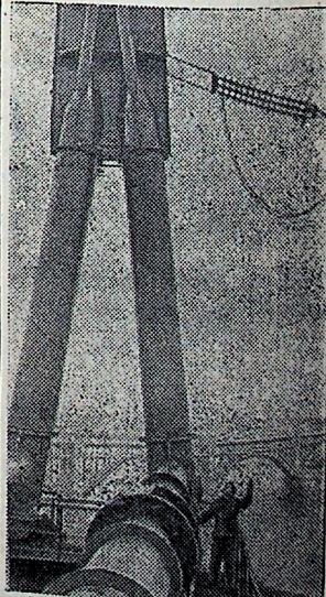
Снимок сделан в момент, когда заканчивался монтаж проводов высоковольтной линии электропередачи Запорожье — Николаев на напряжение 330 киловольт. Скоро по этим проводам, переброшенным через Днепр с помощью высоковольтных мачт, пойдет электрический ток. Фотохроника ТАСС.
