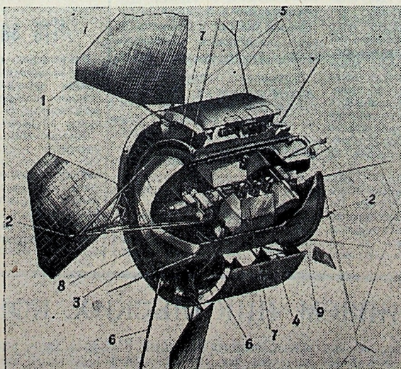
На снимках (слева): Рисунок космической научной станции «Протон-1». Цифрами обозначены: 1—панели солнечной энергетической установки; 2—датчики индикации положения осей станции в пространстве; 3—герметичный корпус; 4—внешняя оболочка; 5—антенны телеметрического, радиокомандного комплекса и
