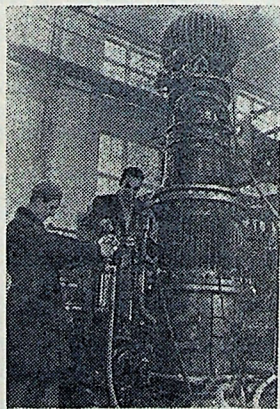
Москва. На экспериментальном электромеханическом заводе Всесоюзного института имени Ленина изготовлены первые специальные ртутные высоковольтные выпрямители. Это оборудование предназначено для линий электропередач постоянного тока напряжением до 500 тысяч вольт. Этот способ передачи энергии на большие расстояния имеет ряд преимуществ. На снимке: электроракумщик Григорий Вобков (слева) и начальник участка сборник Гранат Давтян проверяют вакуумную плотность привода высоковольтного ртутного выпрямителя. Фото В. Кунова. Фотохроника ТАСС.
