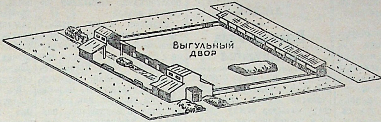
Схема телятника с двумя групповыми автопоилками, выгульным двором, наземным силосным буртом и кормушками для грубых кормов.
