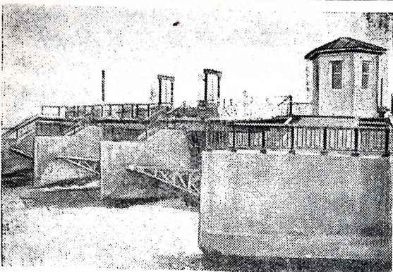
Киргизская ССР. Завершается строительство Большого Чуйского канала. В комплексе с высокогорным Орто-Токойским водохранилищем канал вскоре орошит 60 тысяч гектаров земли, а в дальнейшем зона его действия превысит 100 тысяч гектаров.
