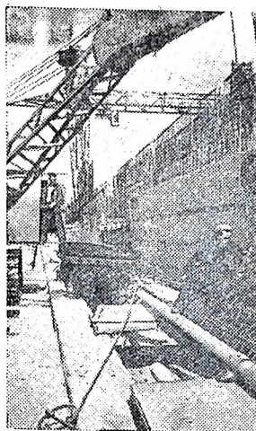
Строительство Воронежской атомной электростанции. Монтаж арматуры. Фото А. Зенина. Фотохроника ТАСС.
