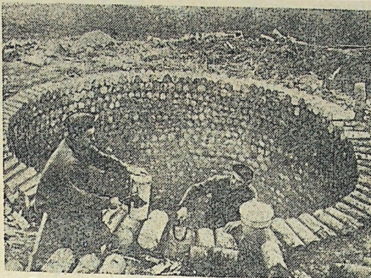
По предложению кузнеца-рационализатора А. А. Голубкова в колхозе «Красный луч» Кубено-Озерского района облицовка силосной ямы на 50 тонн производится осиновыми круглыми чурками. Боковые проемы между чурками замазываются глиняным раствором, а дно и верх торцевой стенки — цементируются. Стоимости сооружения не дороже 2 тысяч рублей.
