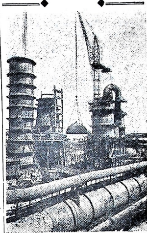
Днепродзержинск. На заводе имени Дзержинского сооружается мощная доменная печь № 12. Она будет работать на повышенном давлении газа под колосником. Коллектив треста «Дзержинскстрой» обязался построить доменную печь со всеми вспомогательными агрегатами в короткий срок — за шесть месяцев. Выполняя взятые обязательства, строители значительно опережают график монтажных работ.
