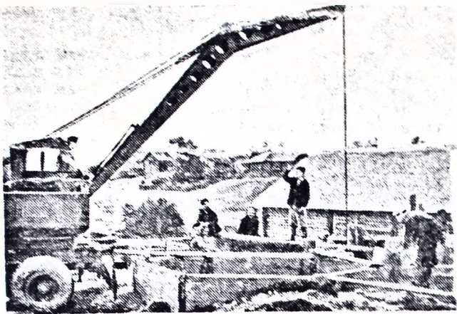
В колхозе «Память Ленина», Лежского района, завершается строительство железобетонной пятисекционной силосной башни на 125 тонн. Строительство ведет колхозная строительная бригада И. А. Корпусова. На снимке: общий вид строительства. В центре бригадир И. А. Корпусов.
