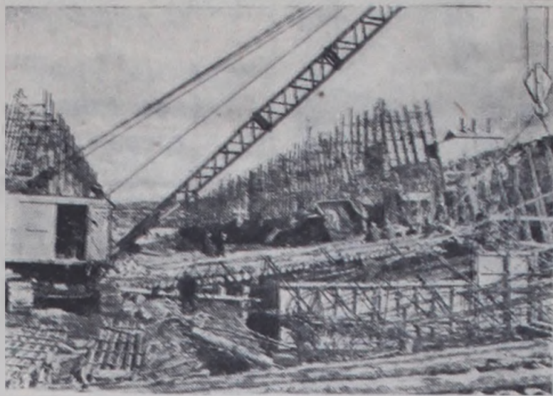
На участках и объектах нового Волга-Тотмисского водного пути сейчас ведутся строительные работы. Сооружается плуза № 2. Из котлована его полностью вынут грунт. С бетонного завода, который недавно смонтирован, в котлован непрерывно поступает бетон и насосами подается в башки шлюза.
