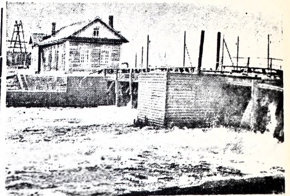
В конце прошлого года на реке Андома была построена и сдана в эксплуатацию межколхозная Князевская ГЭС мощностью 180 киловатт.
