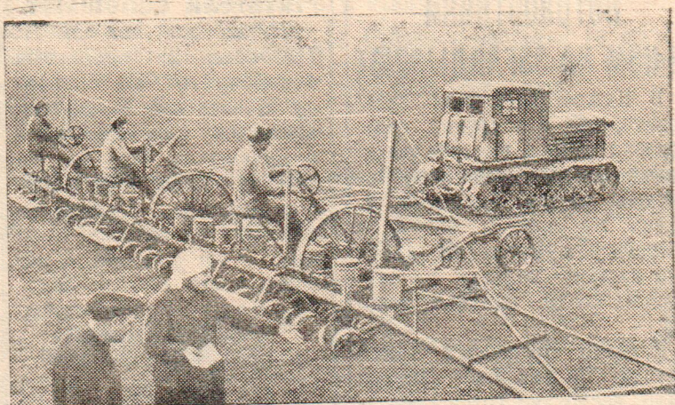
На снимке: посев кукурузы агрегатом из трех сеялок «СШ-6А» на полях колхоза имени Сталина, Ставропольского края. Фото Б. Мясникова и В. Михалева.
