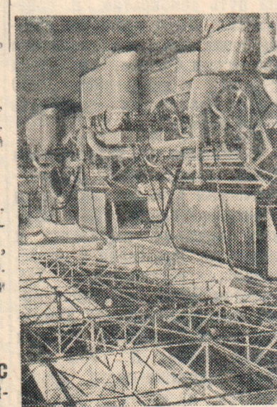
На снимке: большой конвейер сборки хлопкоуборочных машин «СХМ-48м».
