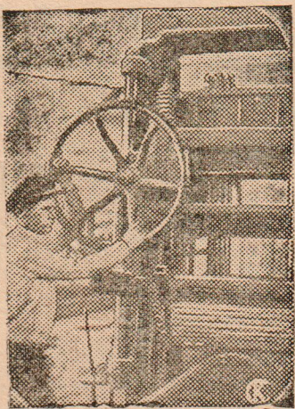
У распиловочной рамы
