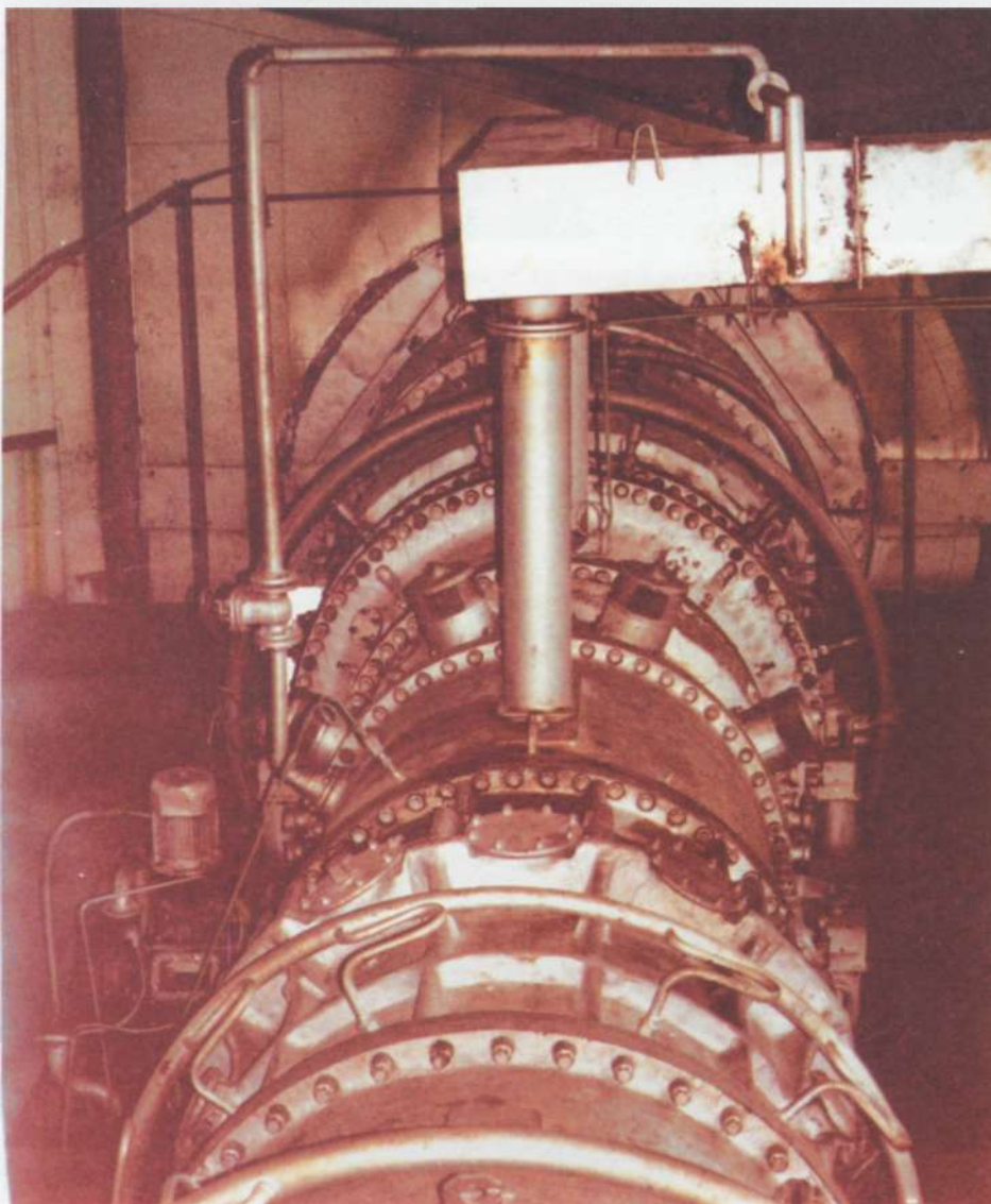
Парогазовая установка на базе ГТН-25/76 и система агрегатной автоматики нового поколения УНК-ГПА на микропроцессорах
