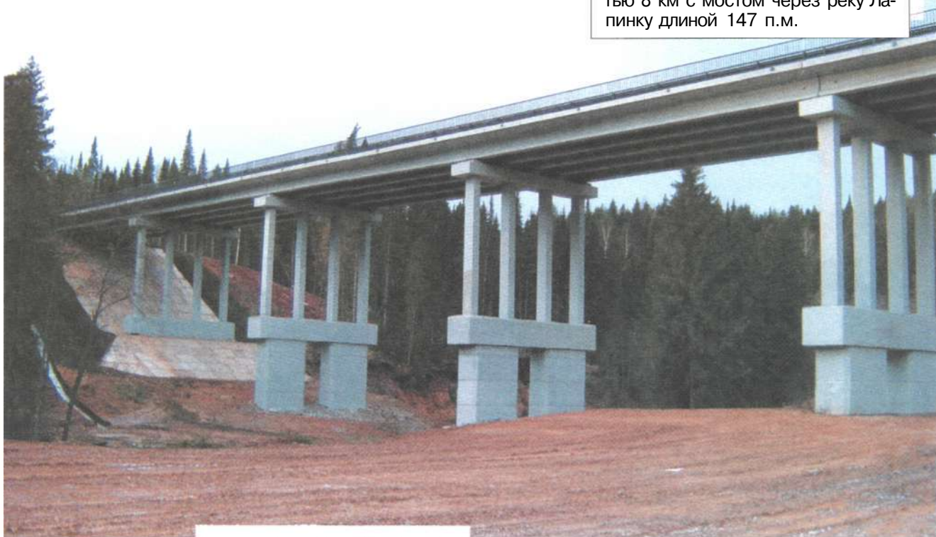
Обход города Красавино, мост через реку Лапинку.
