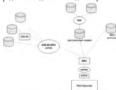
Рис. 4. Архитектура библиотечной сети проекта TEL
