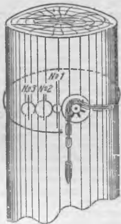
Рис. 2. Схема приростомера системы доц. П. Г. Кроткевича
