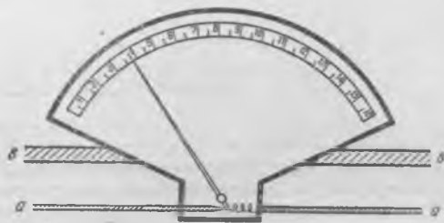
Рис. 1. Схема приростомера сист. проф. Д. И. Товстолеся
