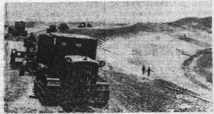
Азербайджанская ССР. В Нахичеванском районе у селения Узуноба сооружается большое водохранилище. Закованная в бетон земляная плотина высотой 18 метров перекроет горное ущелье и образует котлован, который будет заполнен водами реки Нахичеван-чай. Новое сооружение позволит оросить 10 тысяч гектаров земель.
