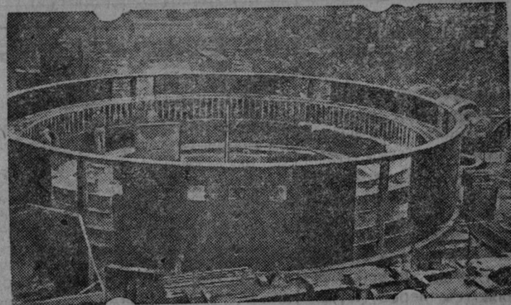
Стахановцы турбинного цеха «Электросила» им. С. М. Кирова (Ленинград) обязались в подарок XVIII съезду ВКП(б) собрать гидрогенератор в 55 тысяч киловатт для Рыбинского гидроузла. На снимке: общий вид собираемого статора машины. Фото Мазолева Бюро-клише ТАСС
