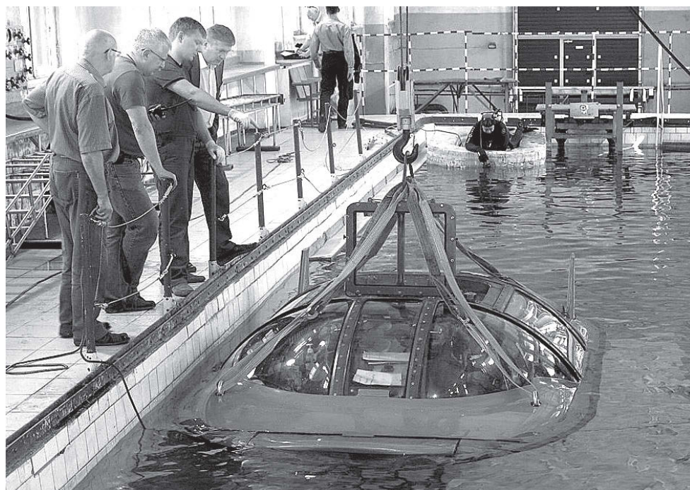
Тренировочный спуск глубоководного аппарата в бассейне.
