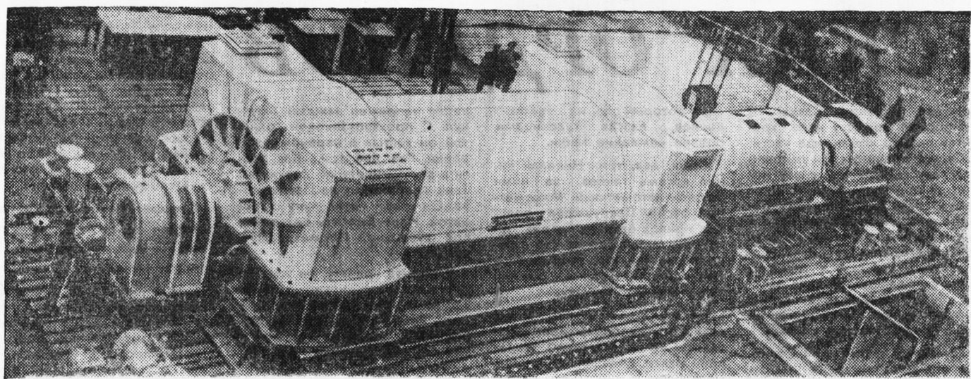
Харьков. На заводе «Электротрактор» имени В. И. Ленина выпущен первый турбогенератор мощностью 500 тысяч киловатт (на снимке). Оригинальная конструкция его разработана инженерами научно-исследовательского института тяжелого электромашиностроения. Созданный в Харькове турбогенератор, охлаждаемый не паром, а водой. Имеет мощность на двести тысяч киловатт больше, чем серийный турбогенератор в 300 тысяч киловатт, новая машина по общему весу на пятнадцать тонн легче, а по габаритам — такая же. Турбогенератор в полмиллиона киловатт предназначен для Назаровской ГРЭС в Красноярском крае.
