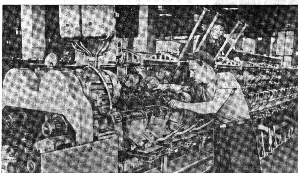
В прядильном производстве Вологодского льнокомбината идет монтаж новых высокопроизводительных машин мягкой мотки. К дню открытия Пленума ЦК КПСС будут смонтированы три такие машины. С применением их ускорится процесс обработки пряжи и улучшится ее качество. На снимке: слесари А. Попов и Н. Кузнецов производят монтаж новой машины. Фото П. Сотникова.
