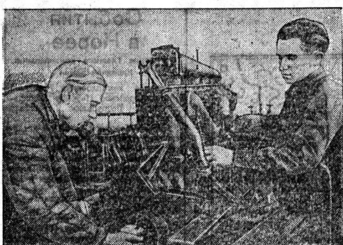
Коллектив Грозненской межрайонной мастерской капитального ремонта дорочно выполнял годовые план и сейчас готовят новые производственные подкаты в честь работников в Верховный Совет РСФСР. На снимке: механик-контролер А. А. Суллов (слева) и слесари-стахановцы П. А. Корюшкин, выполняющий алые свои нормы выработки, за обкаткой и проверкой тракторного мотора на испытательном стенде. Фото П. Сотникова.
