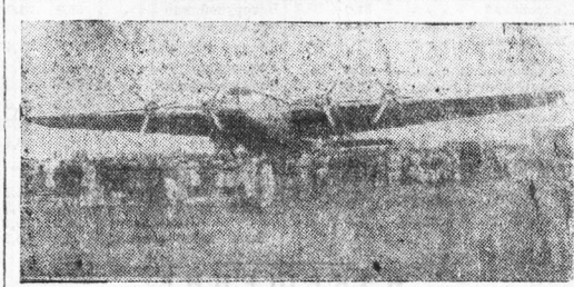
Первый полет самого крупного самолета Англии. Это первый тяжелый самолет из класса 20-тонных «Брайнда». Он имеет скорость 240 км. (150 миль) в час. Наибольшая скорость его более 322 км. (200 миль) в час. Общая длина самолета равна 34 м. 78 см. (114 футов). Размах крыльев достигает 37 метров 52 см. (123 фута). На самолете установлены четыре мотора общей мощностью 3400 лошадиных сил. Внутри самолета может поместиться 42 человека, для которых построены специальные сиденья. На снимке: самолет-гигант на аэродроме. Фото Союзфото.
