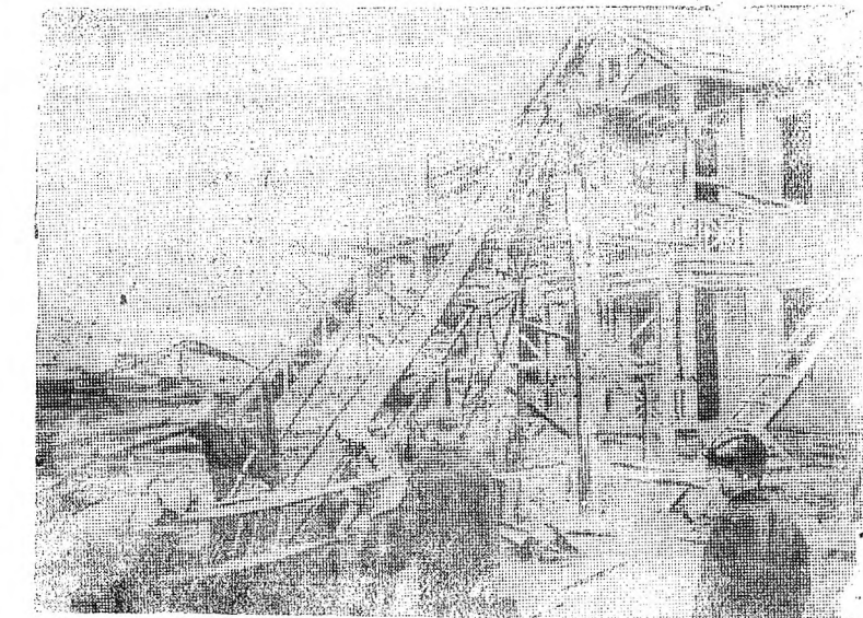
На снимке: Подача стройматериалов электроэлеватором на второй этаж строящегося дома Управления Северной железной дороги на улице Герцена.
