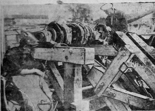
Техжурок завода «Северный коммунар» тов. Маеленикин за монтажем Грузового рабочего вала подъемной фермы плавучего элеватора «СК-2»
