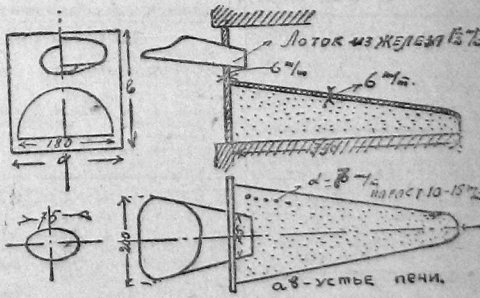
План изобретения тов. Федорова.
