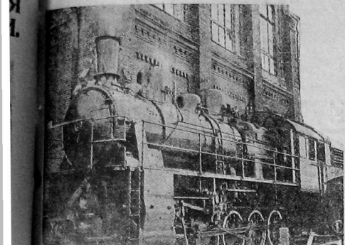
Паровоз № 681-33 выходит на обкатку из паровозного цеха ВРЗ.
