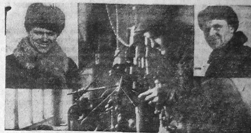
Расшлифовка цилиндров блока автомобильного мотора в гараже ОМЕСа по способу тов. Осминина и Камкина. ВВЕРХУ: СЛЕВА т. ОСМИНИН, СПРАВА т. КАМКИН.
