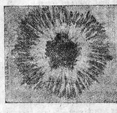
Вид солнечного пятна в сильный телескоп.
