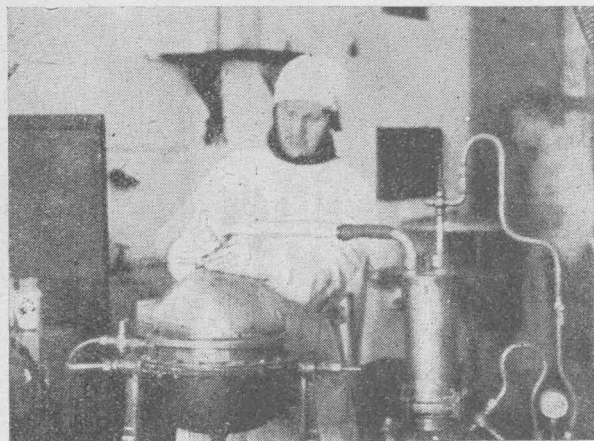
Аппарат «Вакуум».
