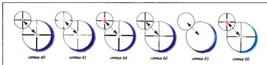
Карл Цейс. Прицельные марки с подсветкой
