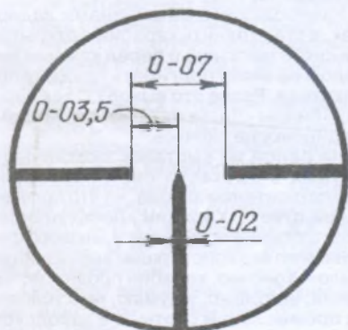
Прицельные нити оптического прицела ПЕ, ТО, ПО
