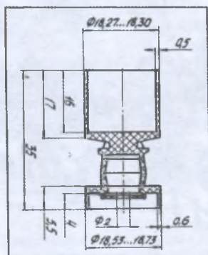
1. Схема пыжа-контейнера фирмы Беретта (Италия)
