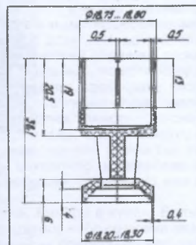
3. Схема пыжа-контейнера фирмы Роттвайл (ФРГ)
