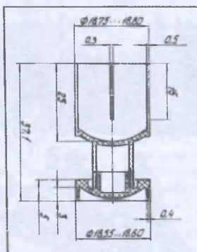
2. Схема пыжа-контейнера фирмы Тунет (Франция)
