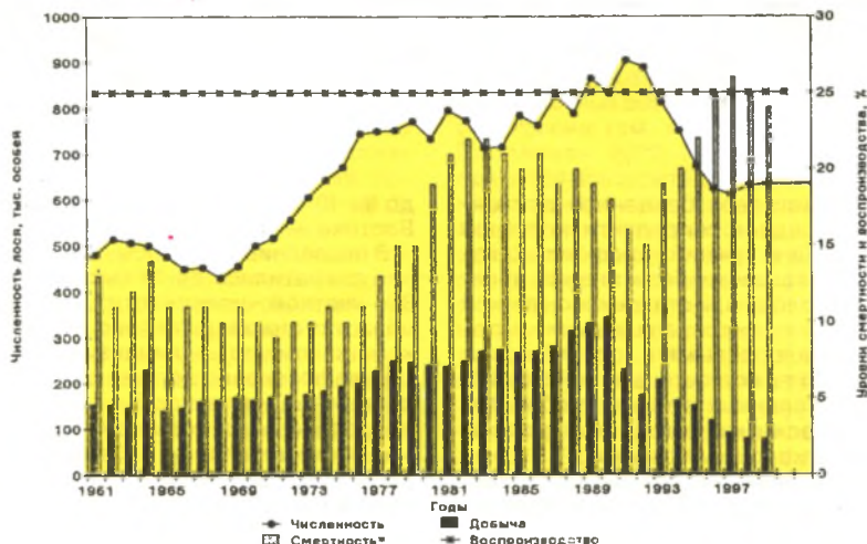
Рис. 1. Динамика численности лосей в зависимости от уровня добычи и хищничества
