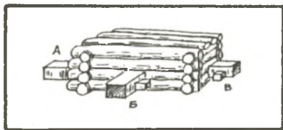
Амбарчик для приваживания соболя: А, Б, В — приставные живоловушки с боковыми утепленными гнездами
