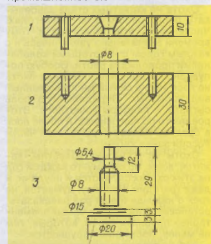
Литейная форма для отливки контейнера: 1 — крышка, 2 — основная пластина, 3 — заготовка под контейнер
