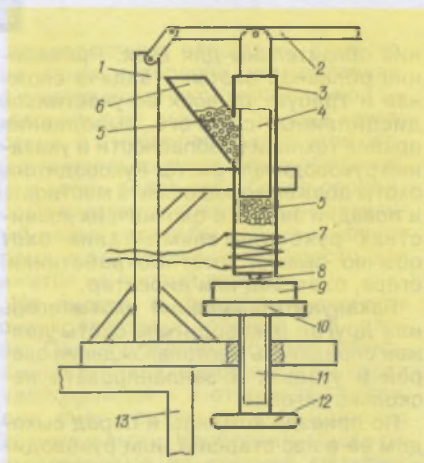
Станок для отливки полиэтиленовых стаканчиков: 1 — рама станка, 2 — рычаг, 3 — рабочий цилиндр, 4 — поршень, 5 — полиэтиленовая крошка, 6 — резервуар для засыпки крошки, 7 — нагревательная спираль на 220 вольт, 8 — заливочный наконечник, 9 — форма, 10 — подставка под форму, 11 — поджимной винт, 12 — штурвал винта, 13 — верстак
