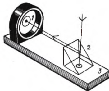
Рис. 1. Схема прохождения световых лучей в коллиматорном прицеле типа «Нидар»: 1 — луч света от неба, 2 — луч, отраженный от марки прицела, 3 — луч, отраженный от основания пирамиды и проектирующий на плоское полупрозрачное стекло марку прицела, которая видна глазу стрелка на фоне местности или цели
