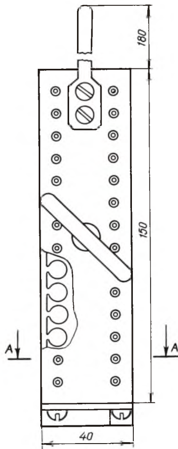
Рис. 1. Литьевая форма
