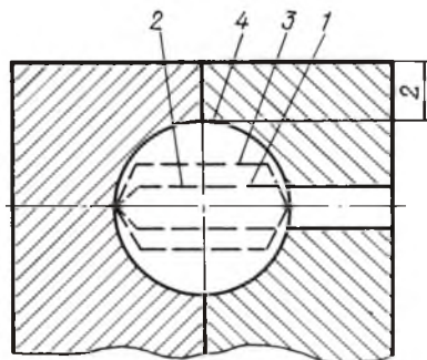
Рис. 2. Порядок сверления полусфер
